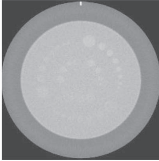
FIG. 32. Low contrast phantom.
